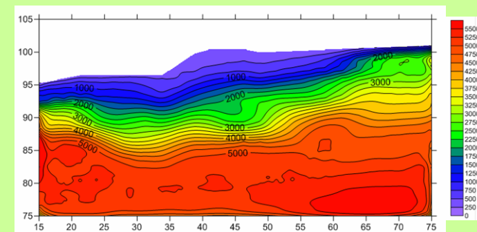
Perfil de Tomografía Sísmica de Refracción
