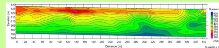
Perfil de Sísmica Masw 2D
